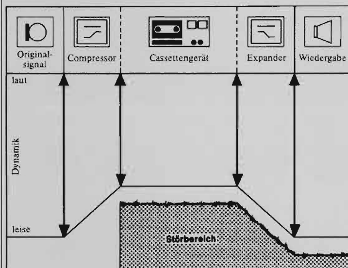
Wirkungsweise des HIGH COM-Rausch- und Störunterdrückungs-Systems
