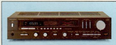
Ⓞ SA-323 UKW/MW-Stereo-Receiver „New-Class-A“-Technik. Raumklangsystem. Ausgangsleistung 2x40 W (Sinus, 4 Ohm). Quarz-Synthesizer-Abstimmsystem mit digitaler Frequenzanzeige. 7 Stationstasten für UKW oder MW. Klirrfaktor 0,007%. LED-Feldstärkeanzeige. Gehäusefarbe: schwarz.
