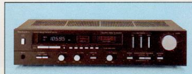
Ⓞ SA-212 UKW/MW-Stereo-Receiver. Ausgangsleistung: 2x30 W (Sinus, 4 Ohm). Quarz-Synth.-Abstimmsystem mit digitaler Frequenzanzeige. 6 Stationstasten für UKW oder MW. Klirrfaktor 0,04%. LED-Feldstärkeanzeige. Gehäuse: schwarz + silber.
