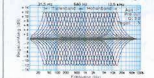
Frequenzgang-Kurven: Einsatzfrequenzen/Schiebereglern
