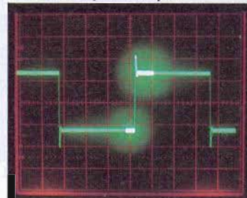
Rechteckverhalten des Nieder-Impedanz-Kopfes
