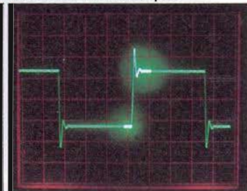
Rechteckverhalten eines konventionellen Kopfes
