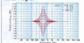
Frequenzgang-Kurven: Level-Regler
