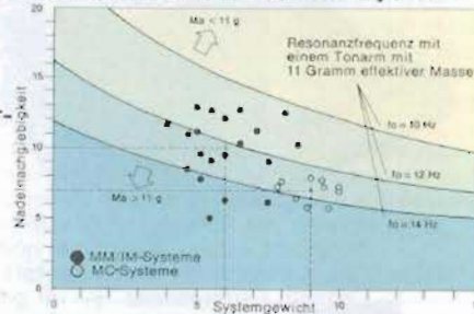
Resonanz-Frequenz des YAMAHA Geraden-Tonarms mit verschiedenen Abtastsystemen
