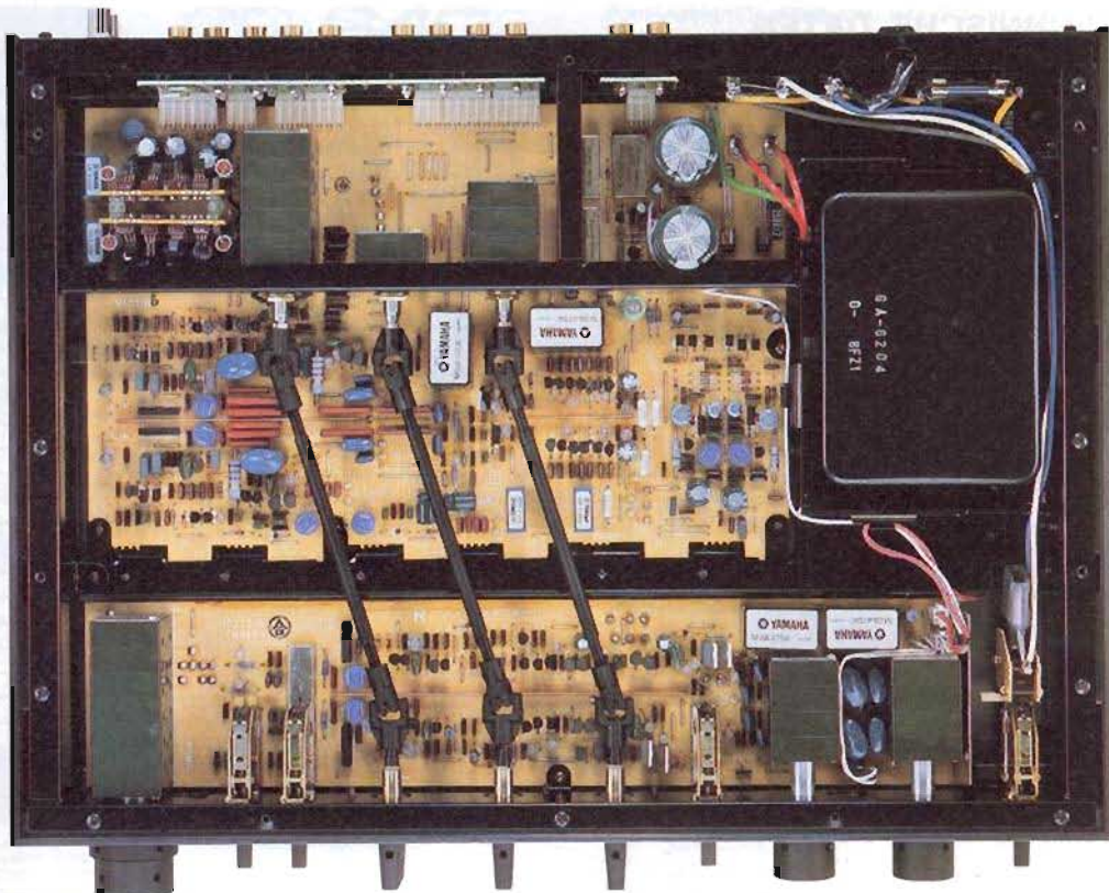
C-2a Innenansicht
