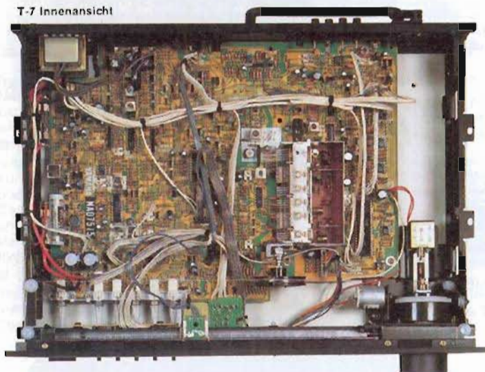
T-7 Innenansicht
