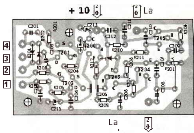
Fig 200.3 – Placa de circuit imprimat 200, dispunerea componentelor, vedere dinspre fața superioară.
