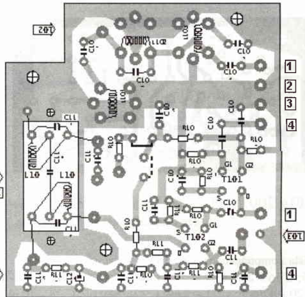
Fig. 100.3 - Placa de circuit imprimat 100, dispunerea componentelor; vedere înspre fața superioară.
