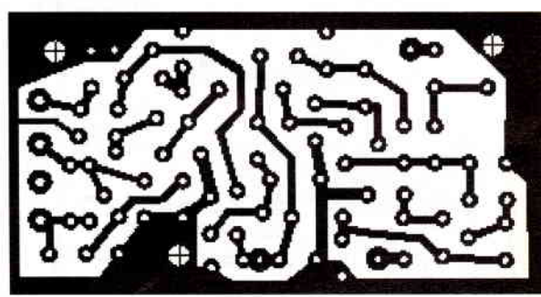
Fig 200.2 – Placa de circuit imprimat 200; vedere dinspre fața inferioară (70 x 37 mm.).
