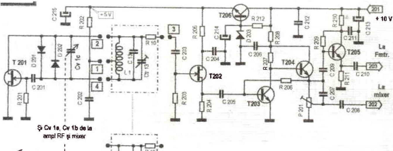
Fig 200.1 – Placa 200; schema primului oscilator local al receptorului.
