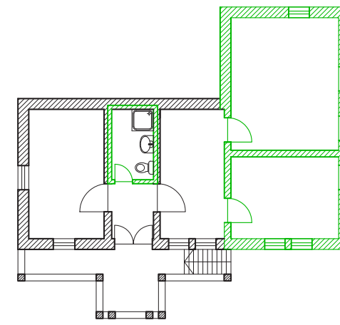
Plan etaj
